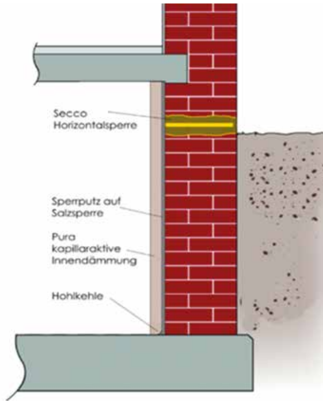
Skizze einer Innenabdichtung.
